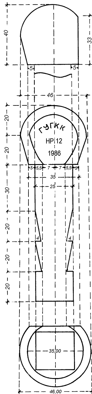
ФОРМА И РАЗМЕРИ НА НИВЕЛАЧЕН БОЛТ М 1:1
