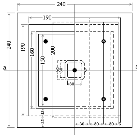
горизонтална проекция
